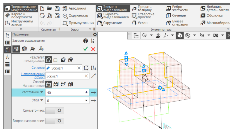
Рисунок 2. Построение фонта объёмного главного вида модели
